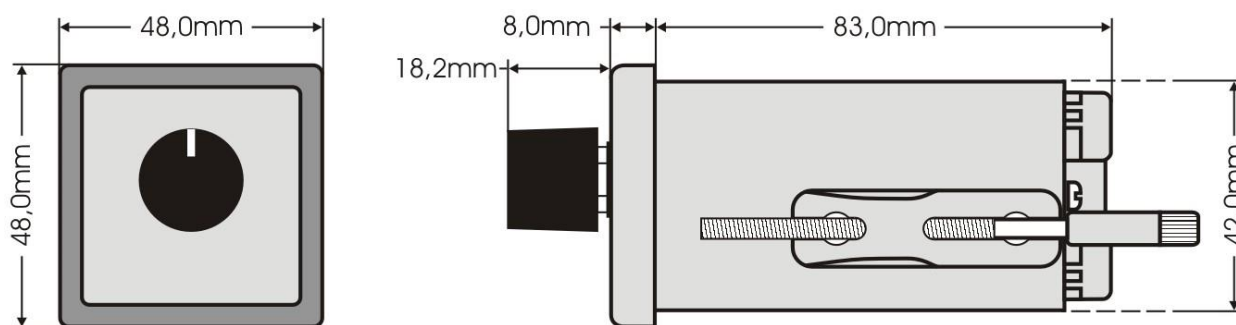
Figura 2: Controlador de Potência Pulsado DIP35.
